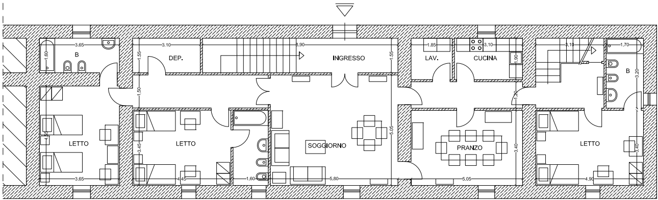
PIANO PRIMO - post operam
